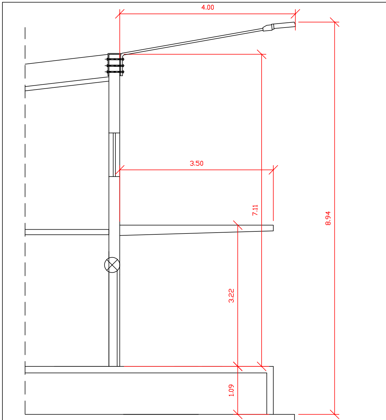
DETALHE PAVILHÃO HF - PARTE MAIOR
