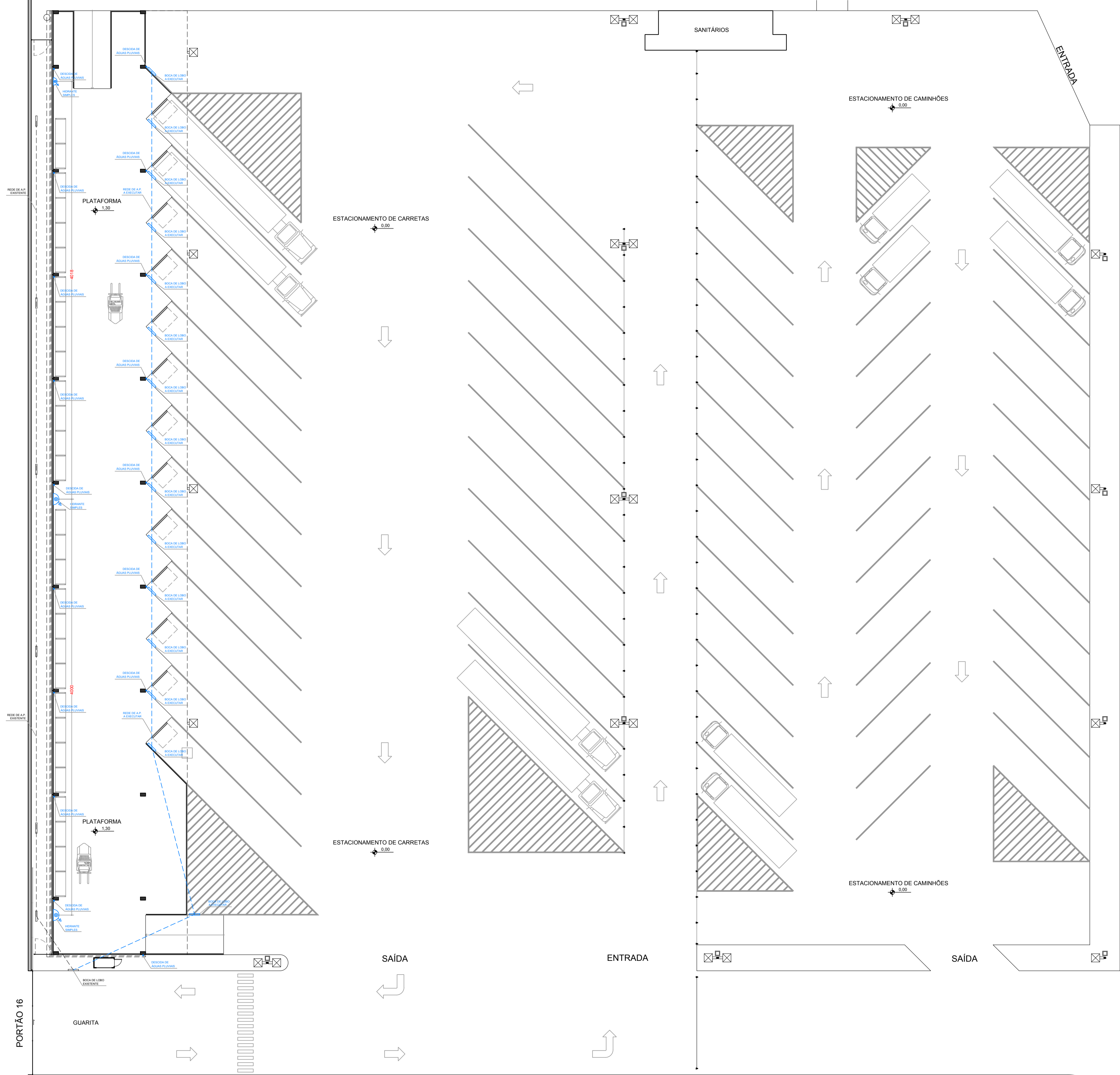
PLANTA DE HIDRÁULICA ESCALA 1:200
