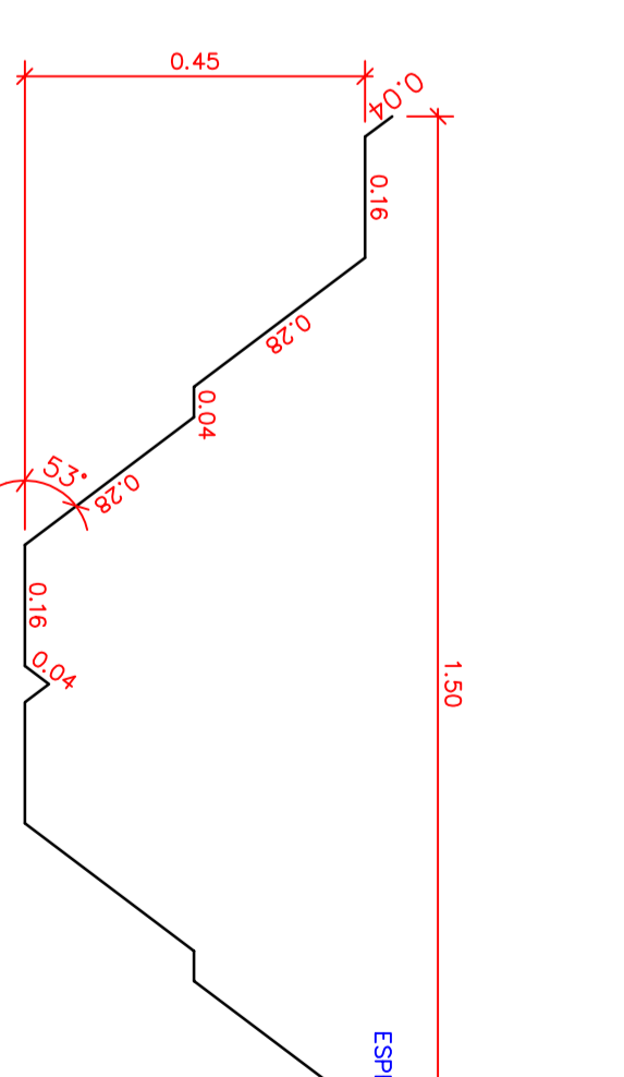
PERFIL DA KP 150 Esc: 1/10
